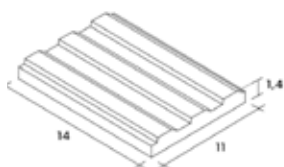
RB 808 14X11
