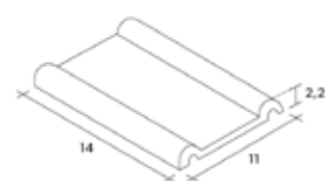
RB 811 14X11
