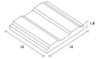
AVRR 20 14X14
