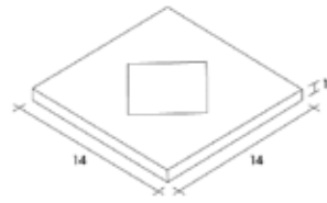
AVRR 13 14X14
