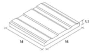
AVRR 22 14X14
